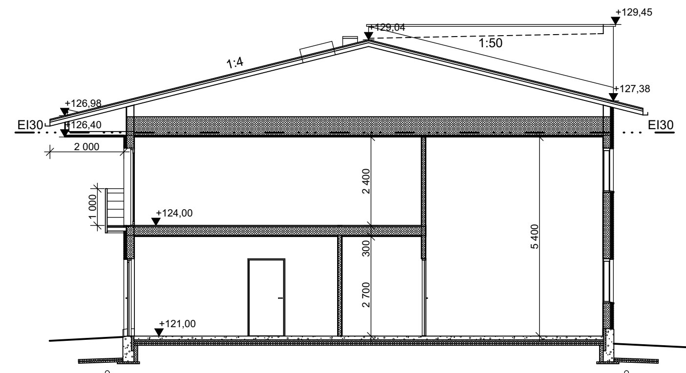
LEIKKAUS A-A
