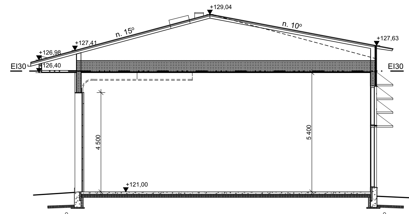
LEIKKAUS B-B
